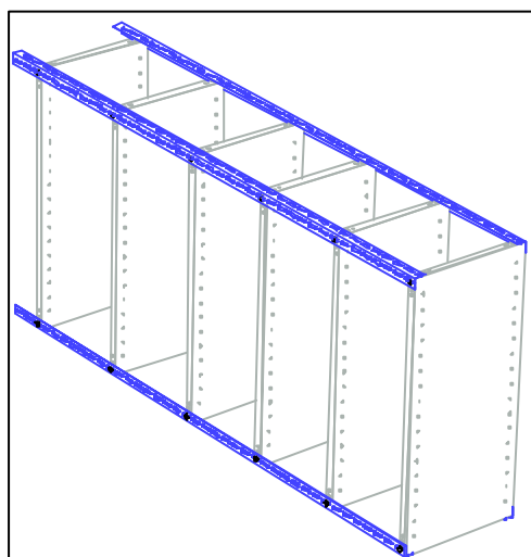
7º Passo: Colocar a 4ª coluna fixando com parafusos e porcas. Manter a lateral da estante sem parafuso e sem porca.
