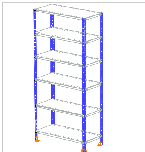
9º Passo: Levantar a estante, montar as demais estantes igualmente para serem unidas posteriormente.
